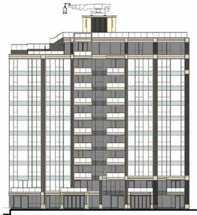
ELEVATION PLAN 1 立面圖 1
