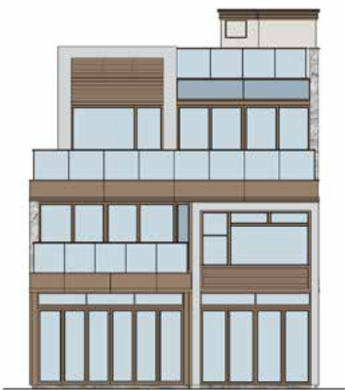
ELEVATION PLAN 1 立面圖 1
